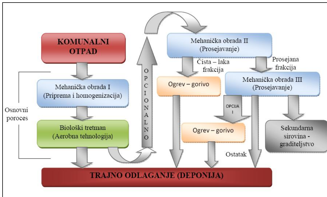
Slika 4.14 Šema MBT tehnologije
