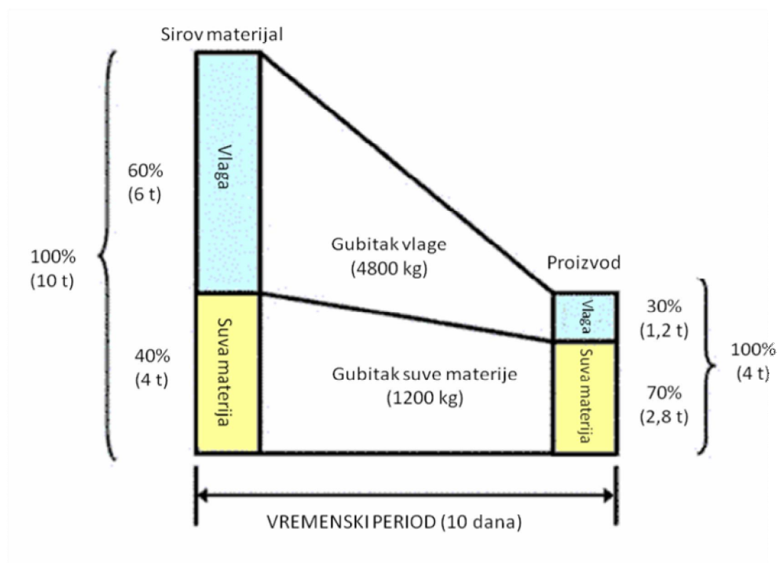
Slika 4.12 Primer procesa kompostiranja
