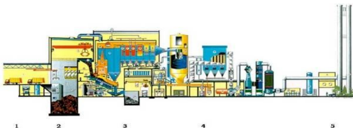
Slika 4.22 Pojednostavljen prikaz postrojenja za insineraciju (1-dopremanje otpada, 2 – Bunker za privremeno skladištenje, 3 – Insineracije, 4 – Sistem za prečišćavanja dimnih gasova, 5 – dimnjak)
