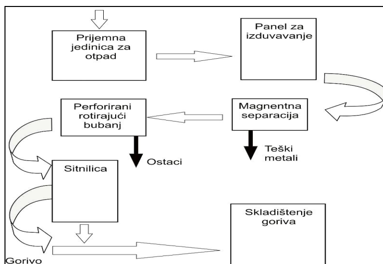
Slika 4.24. Šema proizvodnog procesa goriva dobijenog iz otpada (RDF)
