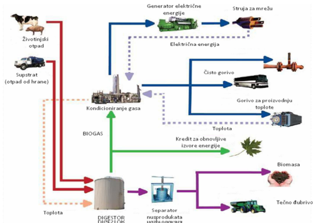
Slika 4.13 Dijagram toka korišćenja produkata procesa anaerobne digestije
